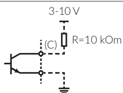
Схема подключения импульсного кабеля
