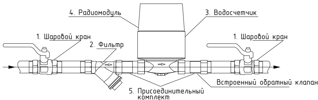
Схема водомерного узла
